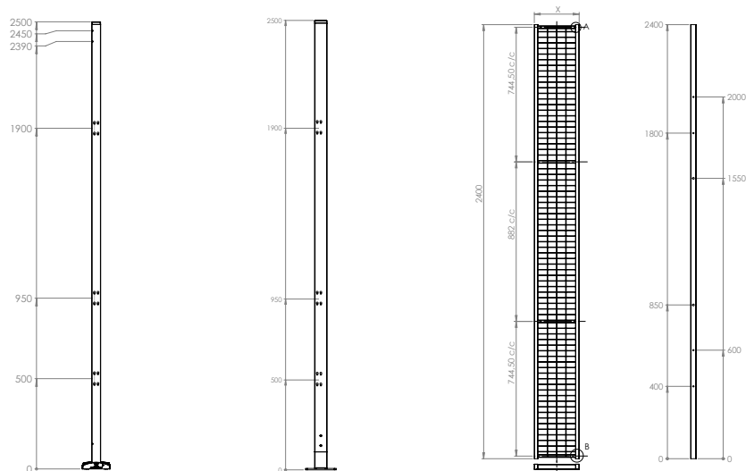
Bodenstützen 50x50 Bodenstützen 70x70
