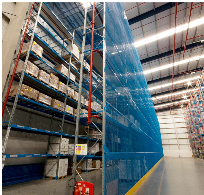
SafeStore-Giterrückwand, 12 Meter hoch, 55 Meter lang, als Teil der Schutzvorkehrungen in einem Aerosollager. Die Ausführung der Giterrückwand erfolgte in Spezialfarbe und mit massiven Elementaufnahmen, um den hohen Anforderungen des Kunden zu entsprechen.
